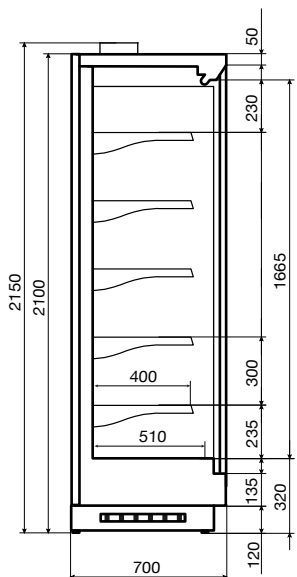
Vega DG 070 H210
