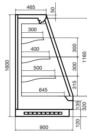
Vega DG 090 H160
