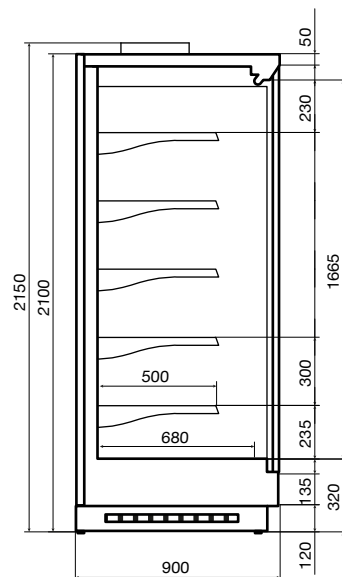
Vega DG 090 H210
