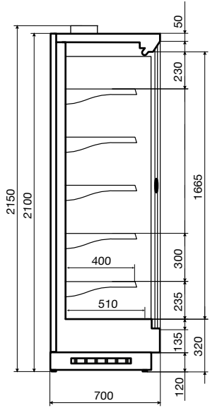
Vega SG 070 H210
