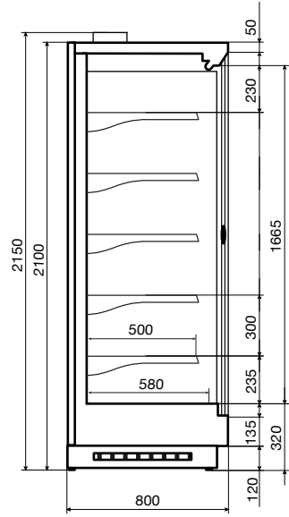
Vega SG 080 H210
