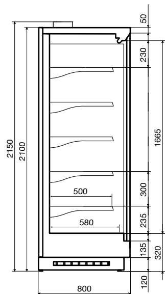
Vega DG 080 H210
