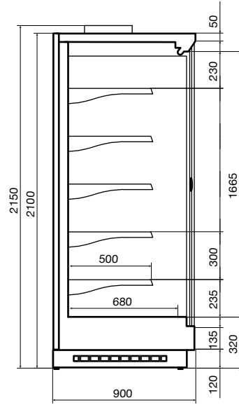
Vega SG 090 H210
